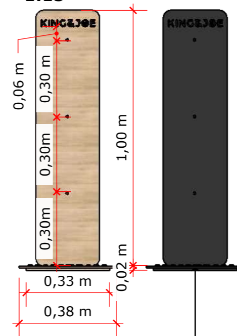
V. F. EXPOSITOR 12 E 13 1:15
