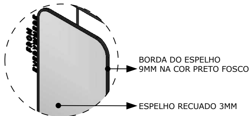
DET. 04 1:10
