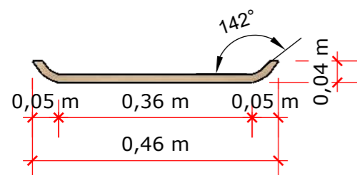
DET. 06 1:10
