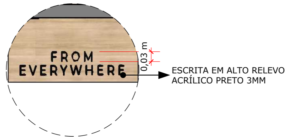
DET. 10 1:7
