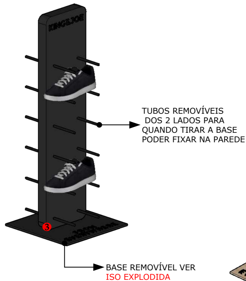
ISO - EXPOSITOR 2 1:10
