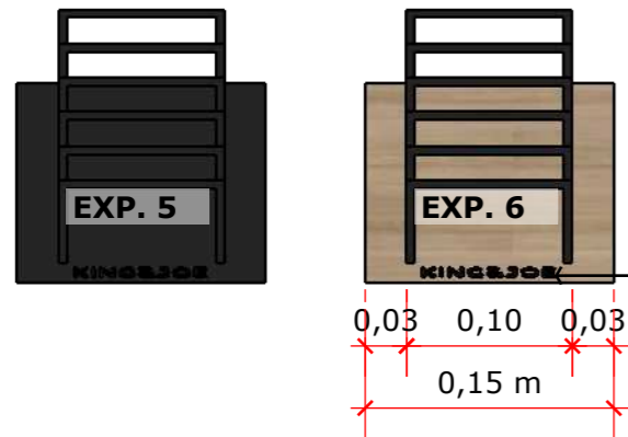
ISO EXPOSITOR 5 E 6 1:5
