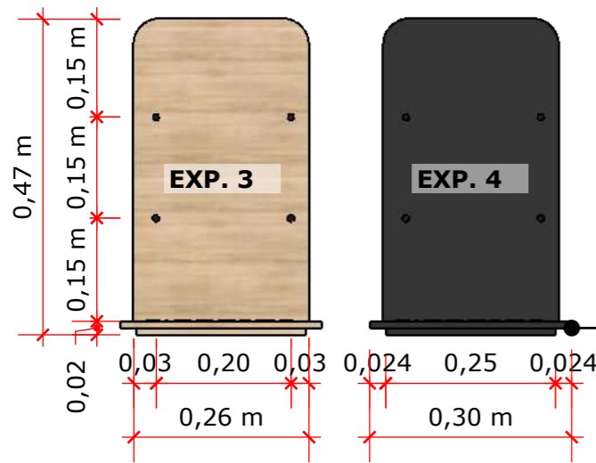
V. F. EXPOSITOR 3 E 4 1:10
