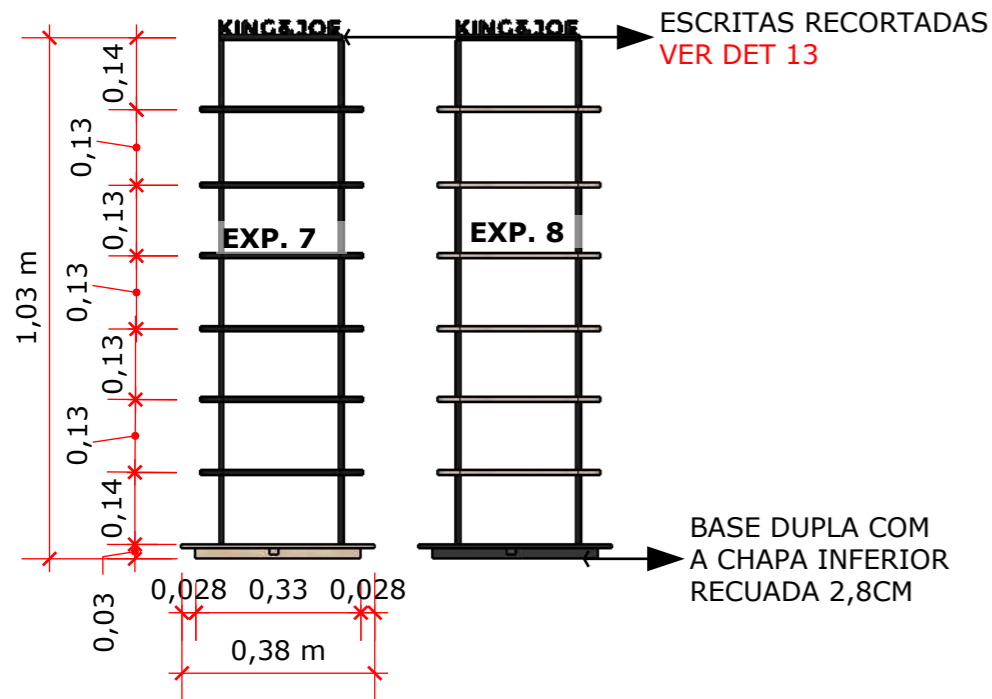
V. F. EXPOSITOR 7 E 8 1:15
