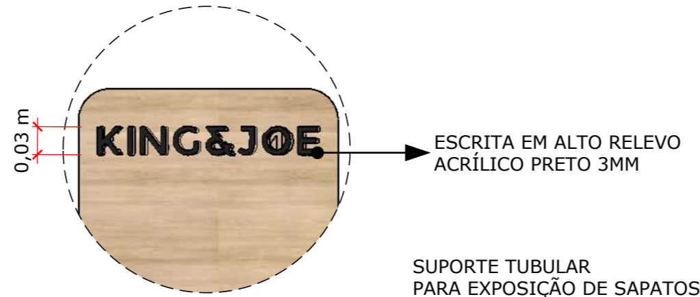
DET. 09 1:5
