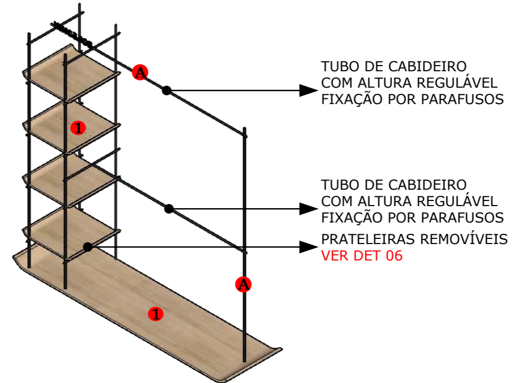
ISO ARARA S/ ESPELHO 1:25
