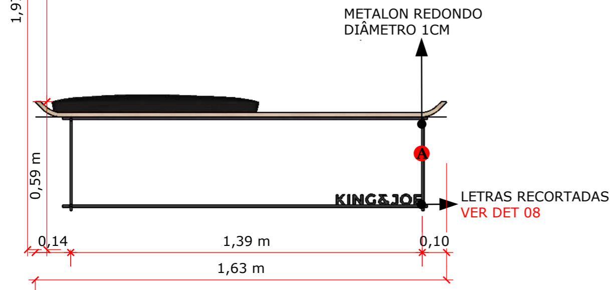
DET. 07 1:10
