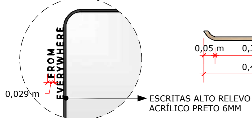
DET. 02 1:10
