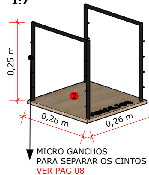
ISO EXPOSITOR 9 1:7
