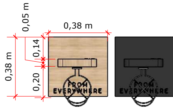
V. S. - EXPOSITOR 10 E 11 1:15
