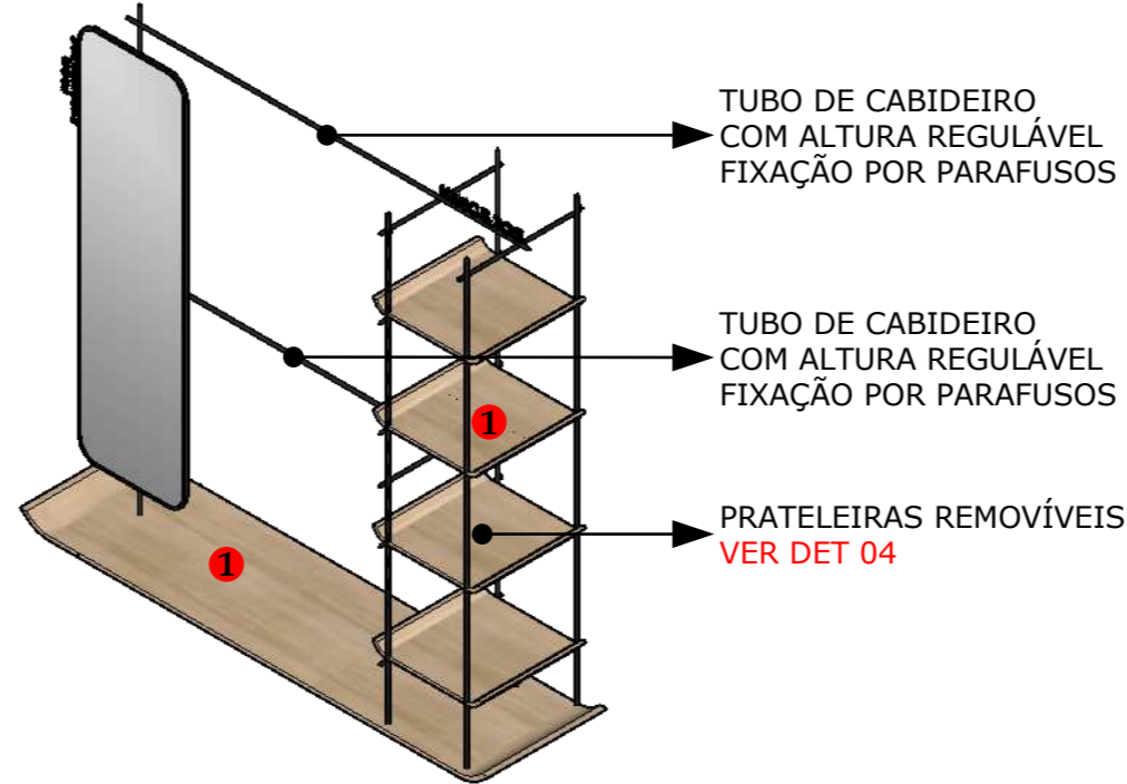
V. P. ARARA ESPELHO 1:25
