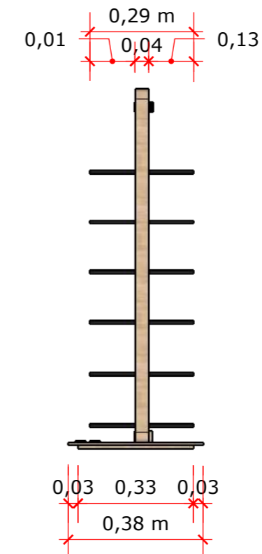
V. L. D. EXPOSITOR 2 1:15
