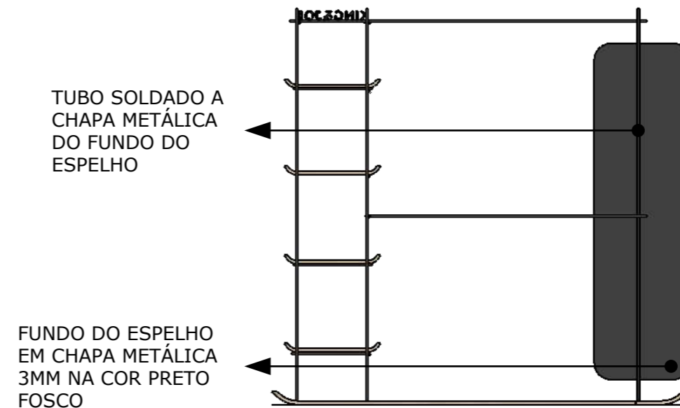
V. P. ARARA ESPELHO 1:25
