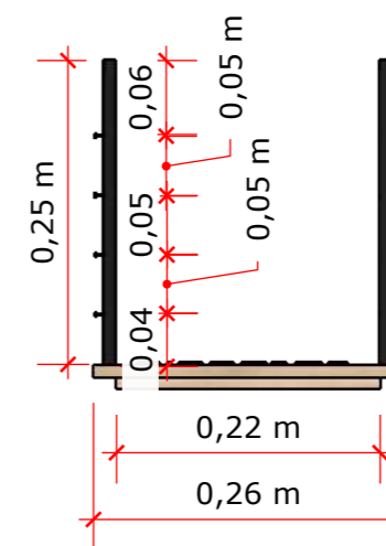
V.F EXPOSITOR 9 1:7
