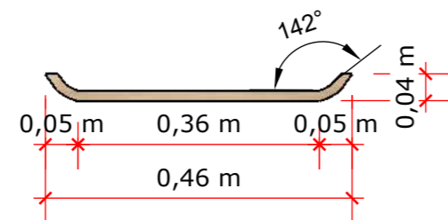
DET. 04 1:10
