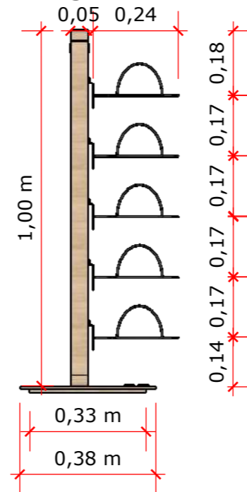
V. L. - EXPOSITOR 10 E 11 1:15
