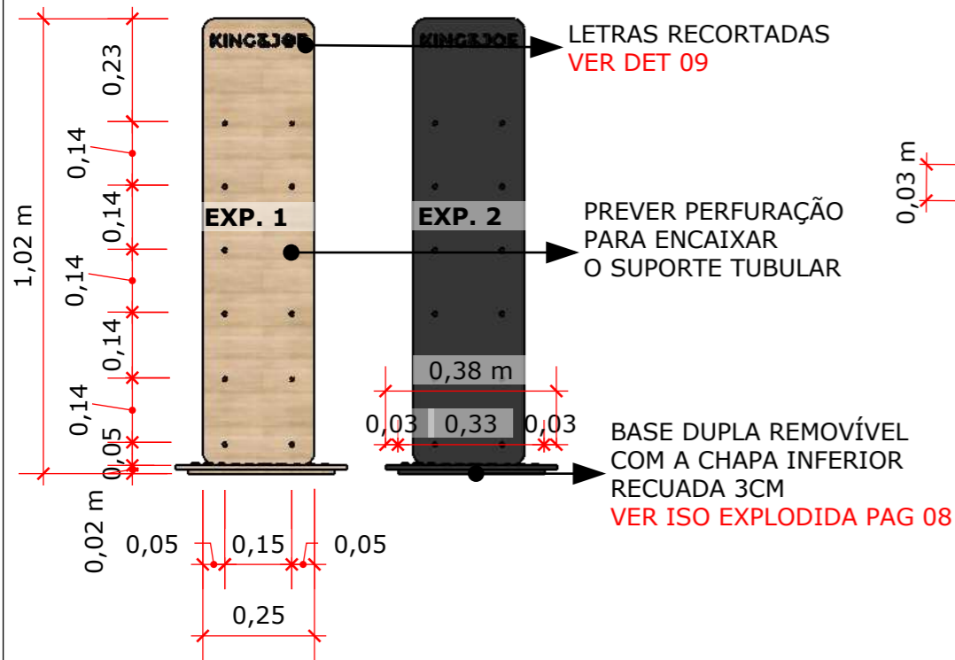
V. F. EXPOSITOR 1 E 2 1:15
