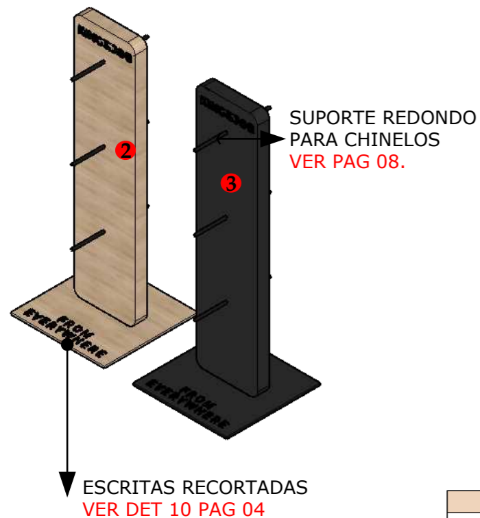
V. F. EXPOSITOR 12 E 13 1:15
