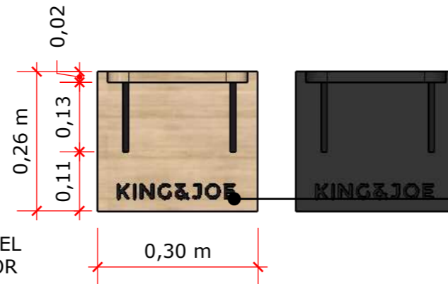
V. S. EXPOSITOR 3 E 4 1:10
