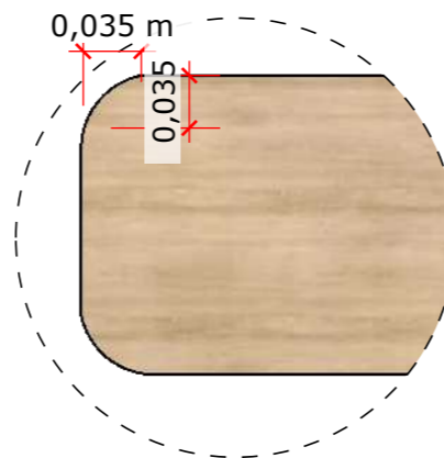
DET. 15 1:5
