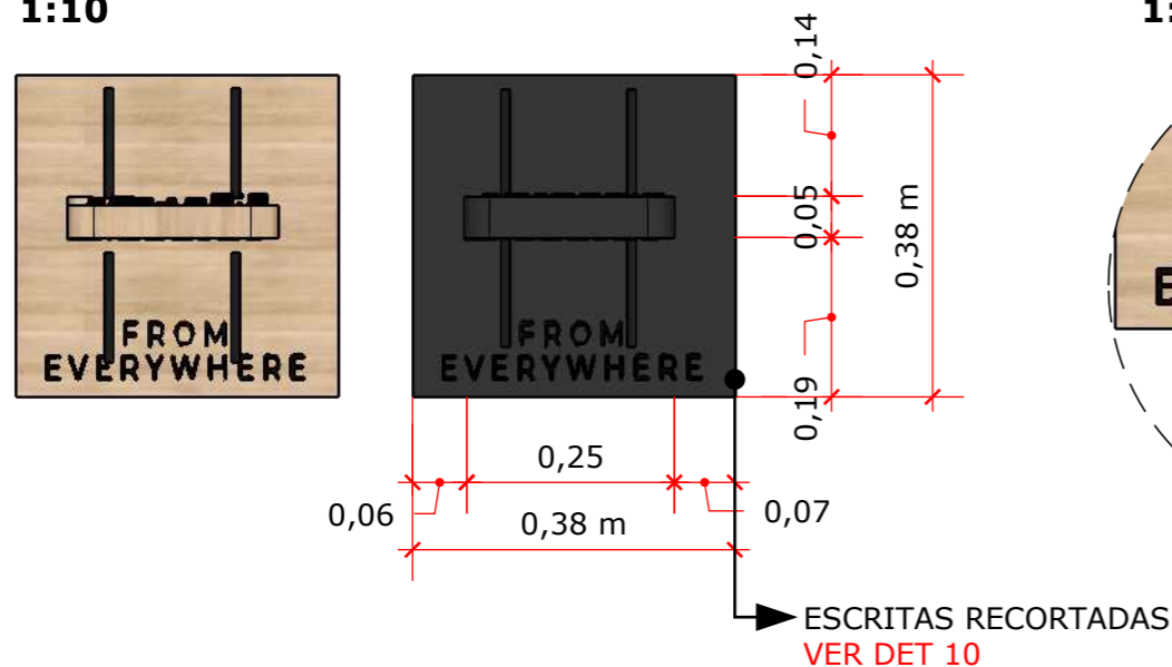
V. S. EXPOSITOR 1 E 2 1:10
