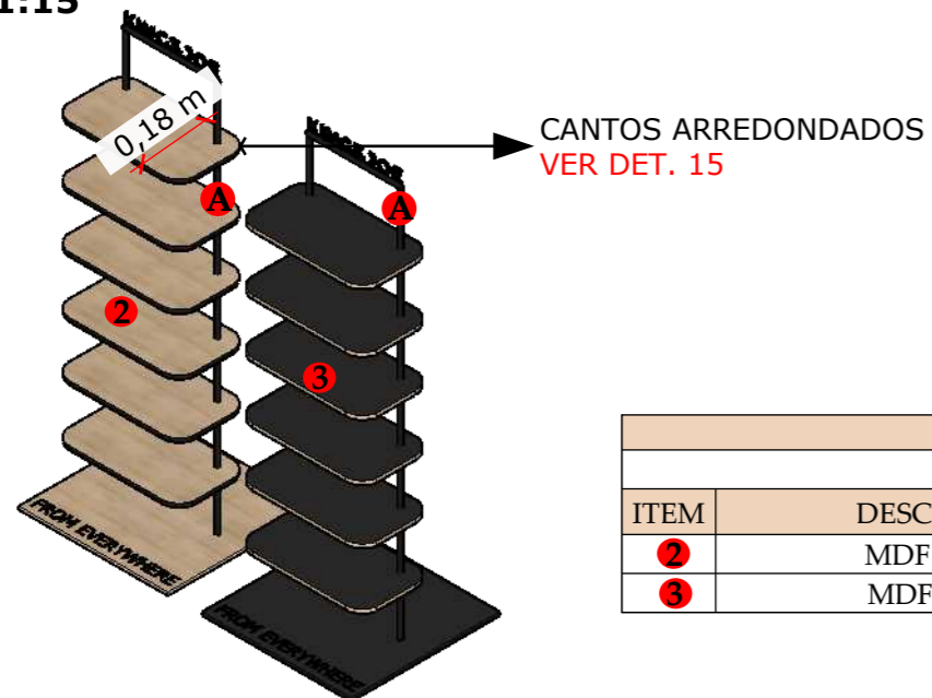
ISO EXPOSITOR 7 E 8 1:15
