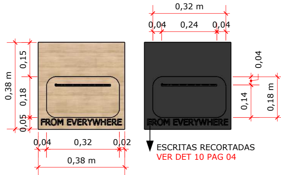
V. S. EXPOSITOR 7 E 8 1:10
