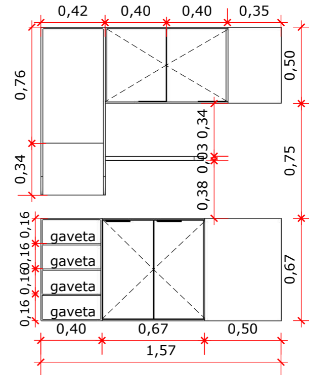
V.L - ARMÁRIOS 1:25
