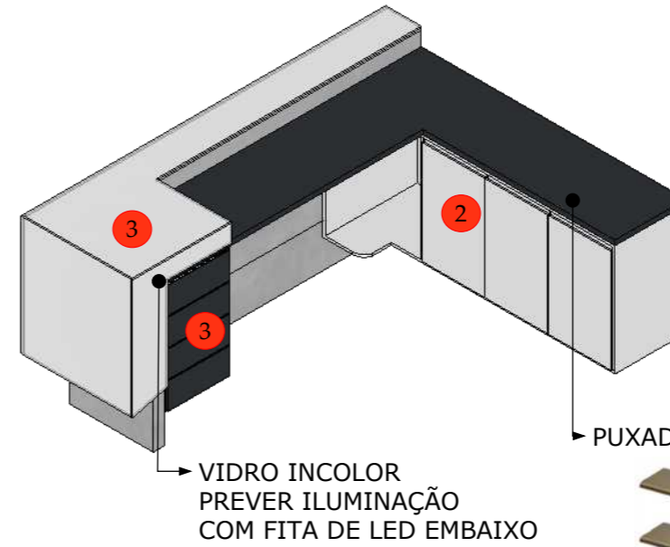
ISO TRÁS - BALCÃO DE ATENDIMENTO 1:30
