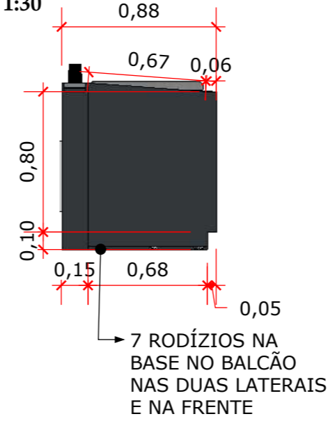
V.L - BALCÃO DE SERVIR 1:30
