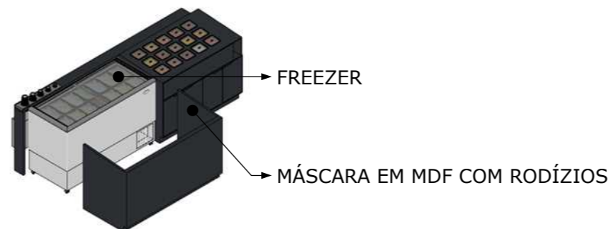
ISO - BALCÃO DE SERVIR - DESMONTADO 1:30
