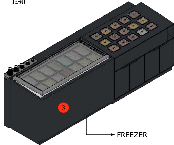
ISO - BALCÃO DE SERVIR 1:30
