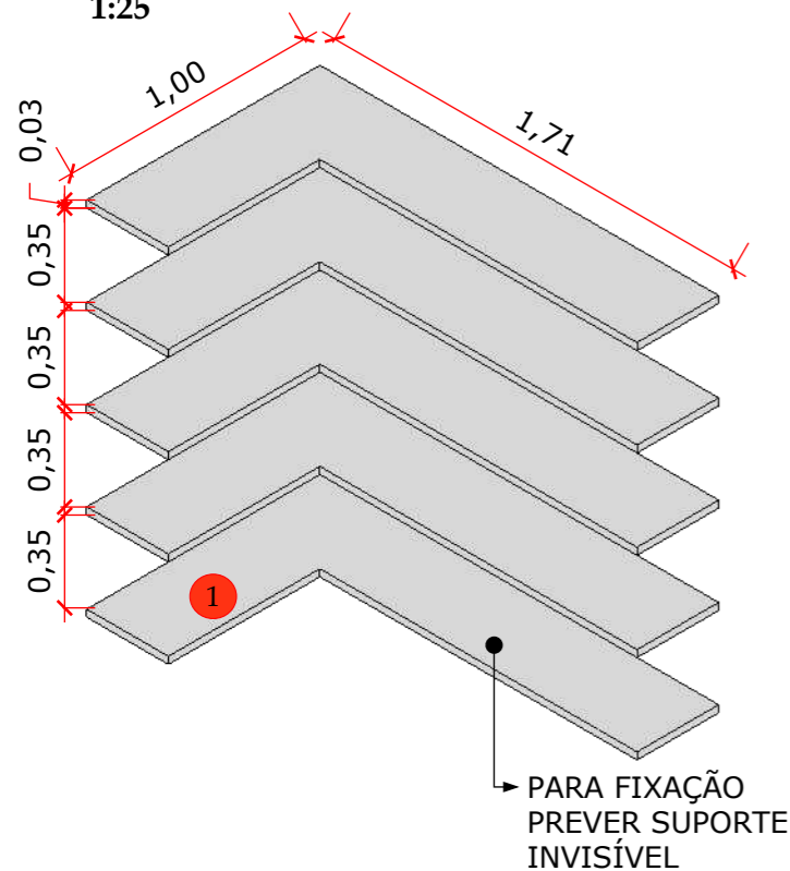
ISO - PRATELEIRAS 1:25
