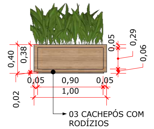
V.F - CACHEPÓ 1:30
