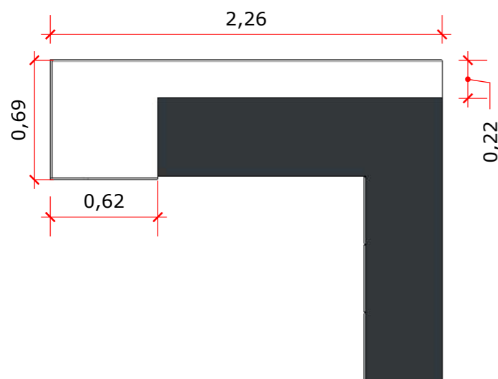
V.S - BALCÃO DE ATENDIMENTO 1:30
