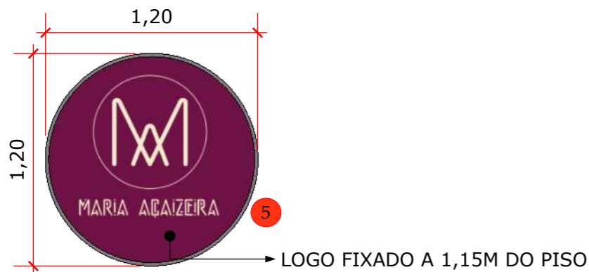
V.F - LOGO 1 1:30
