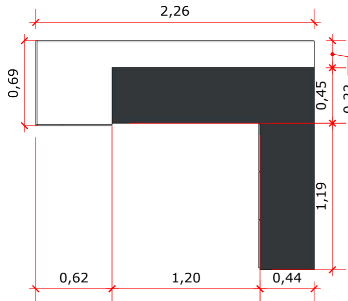
V.S - BALCÃO DE ATENDIMENTO 1:30
