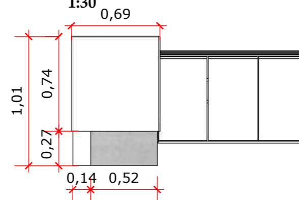
V.L - BALCÃO DE ATENDIMENTO 1:30
