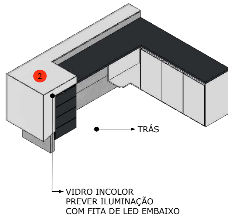
ISO - BALCÃO DE ATENDIMENTO 1:30
