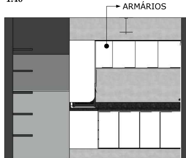
VISTA 2 1:40
