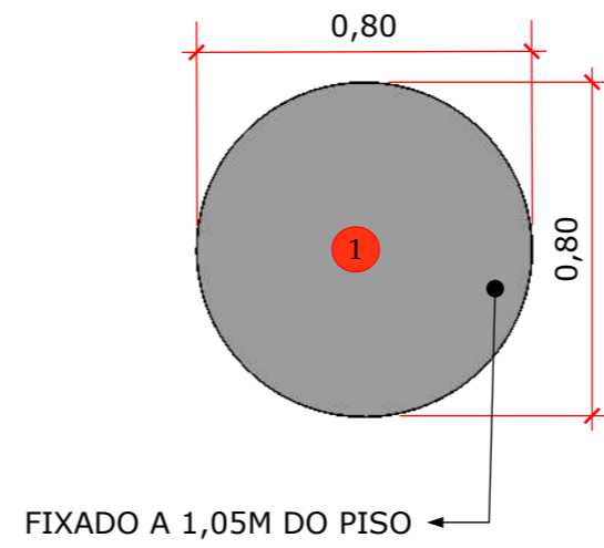
V.F - ESPELHO 1:30
