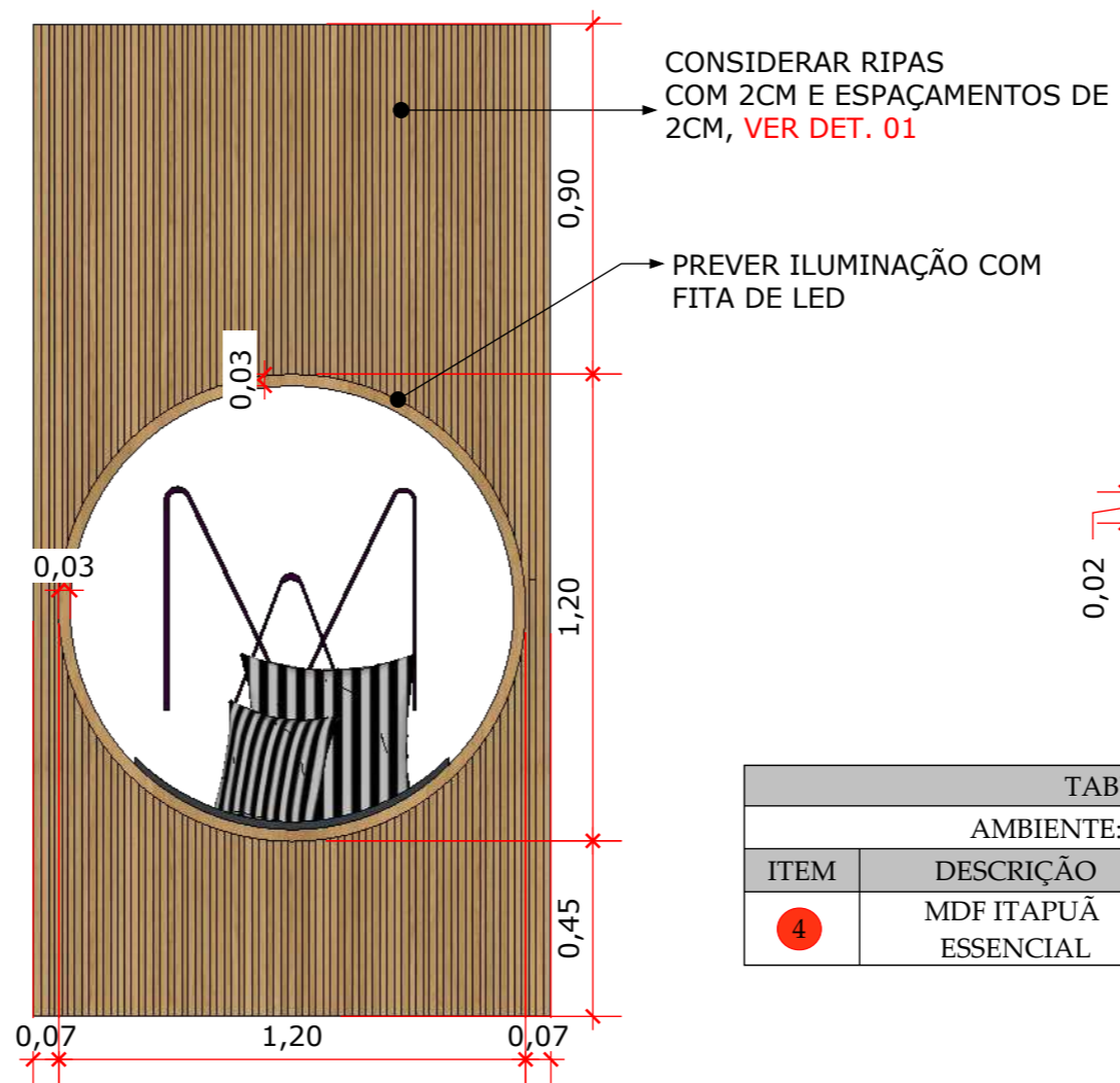
V.F - PAINEL RIPADO 1:20
