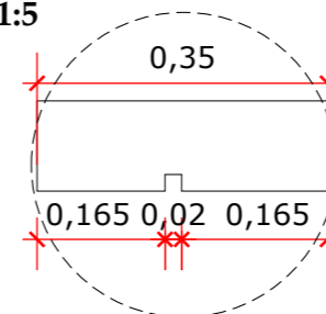
DET. 02 PERFIL DE LED 1:5
