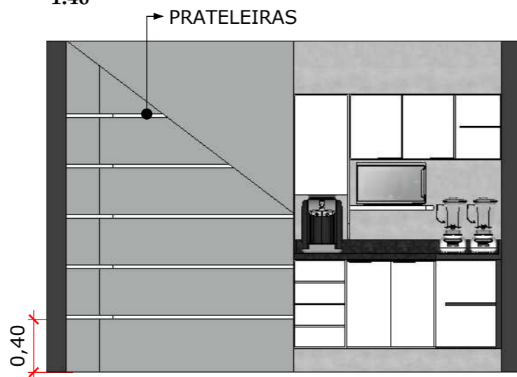
VISTA 1 1:40
