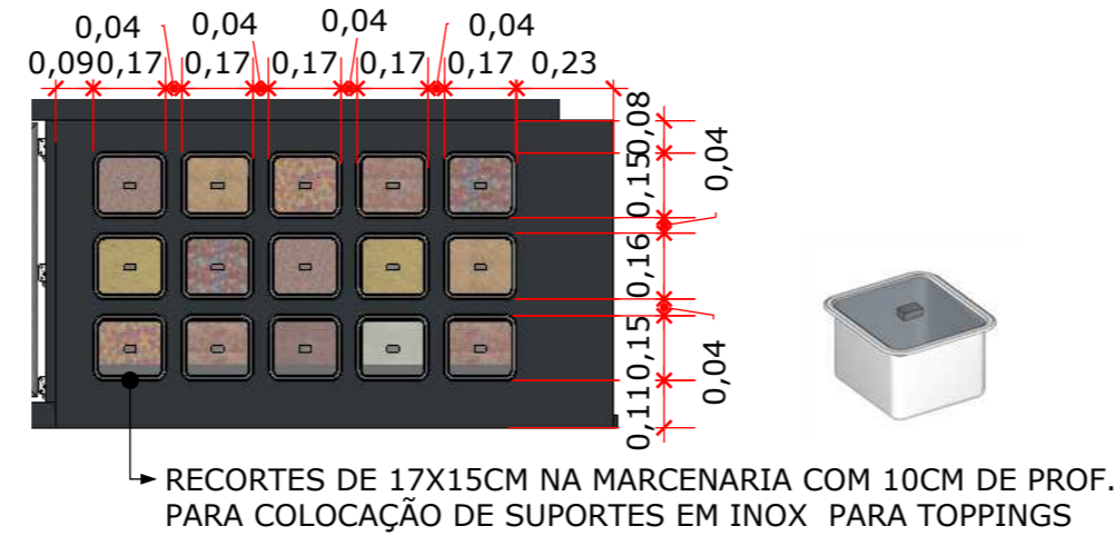
V.S - BALCÃO DE SERVIR TOPPING 1:20
