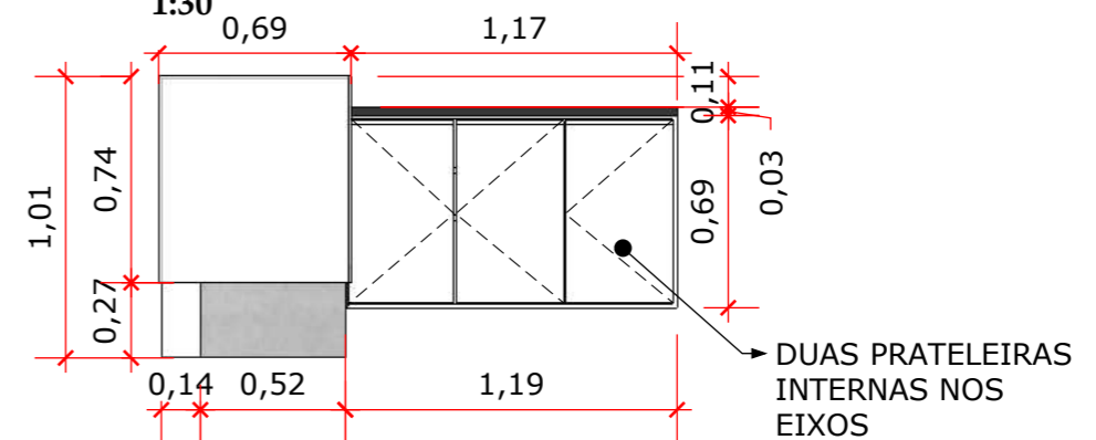
V.L - BALCÃO DE ATENDIMENTO 1:30
