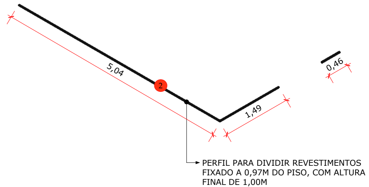
ISO - PERFIL 1:40
