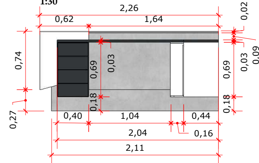
V.L - BALCÃO DE ATENDIMENTO 1:30
