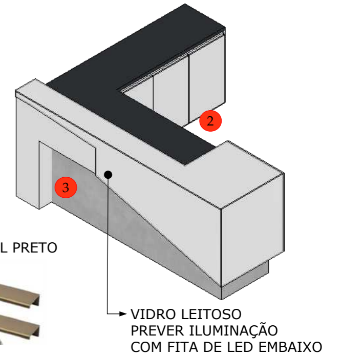
ISO FRENTE - BALCÃO DE ATENDIMENTO 1:30
