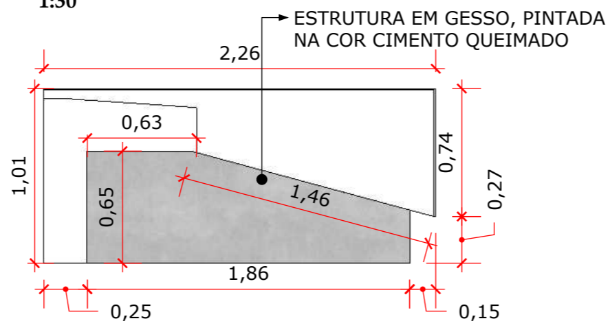
V.F - BALCÃO DE ATENDIMENTO 1:30
