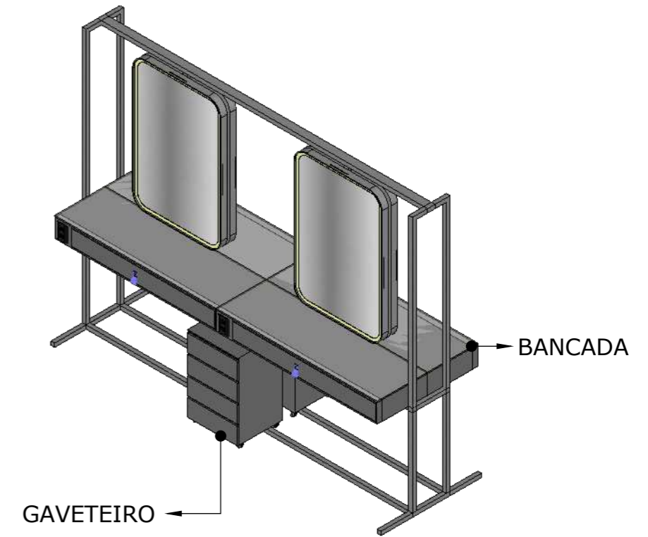
ISO - PENTEADEIRA 1:30
