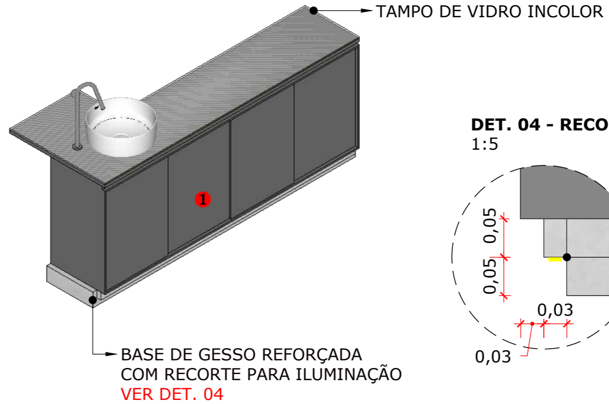
ISO BANCADA 1:20
