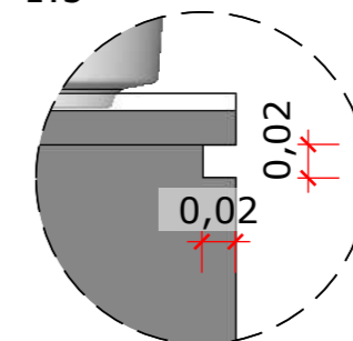
DET. 06 - RECUO MARCENARIA 1:5
