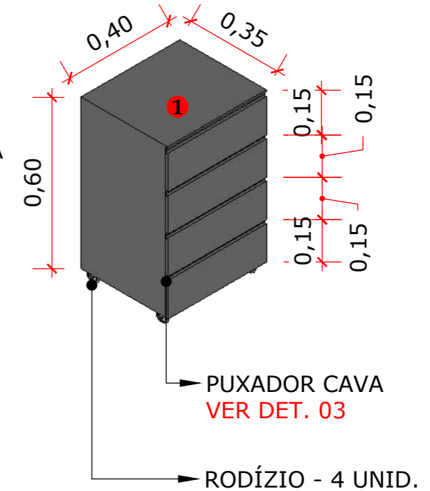
ISO - GAVETEIRO 1:15
