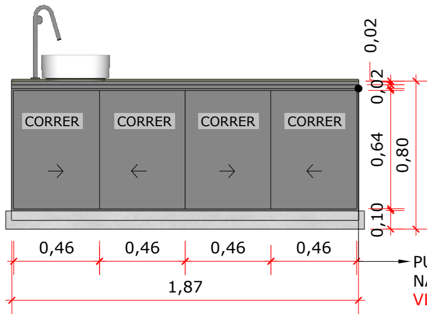
V. F. - BANCADA 1:20
