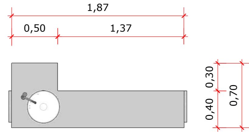
V. S. - TAMPO BANCADA 1:25
