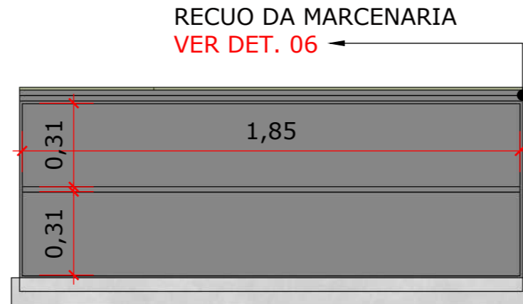
DET. 05 - PUXADOR CAVA 1:3
