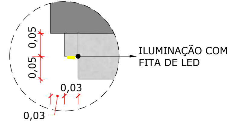
DET. 04 - RECORTE BASE 1:5
