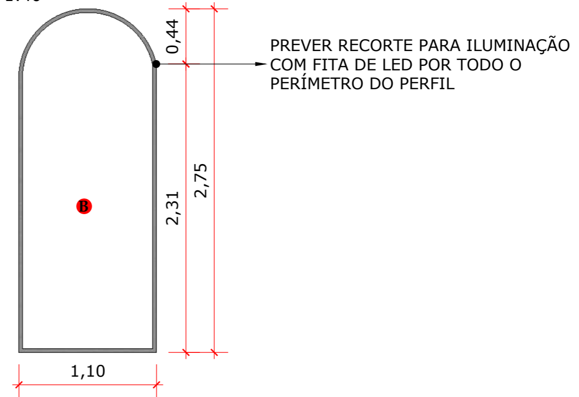
V. F. - MOLDURA PAREDE 1:40
