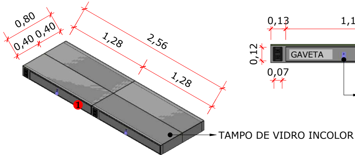
ISO - BANCADA 1:30
