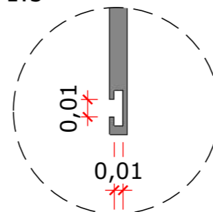
DET. 05 - PUXADOR CAVA 1:3
